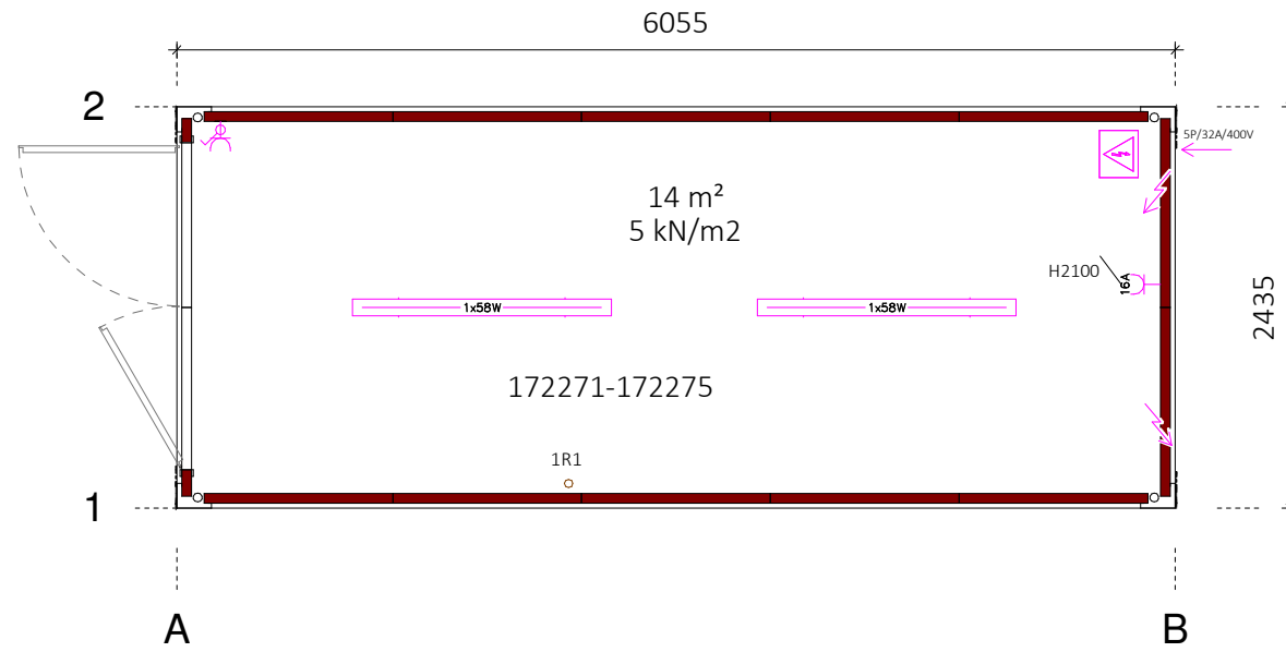
Tloris 1 : 50
