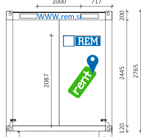
Pogled z desne 1 : 50
