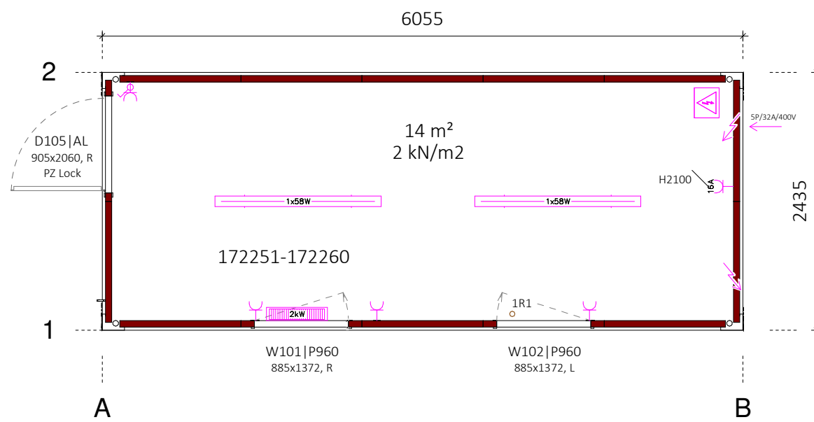
Tloris 1 : 50
