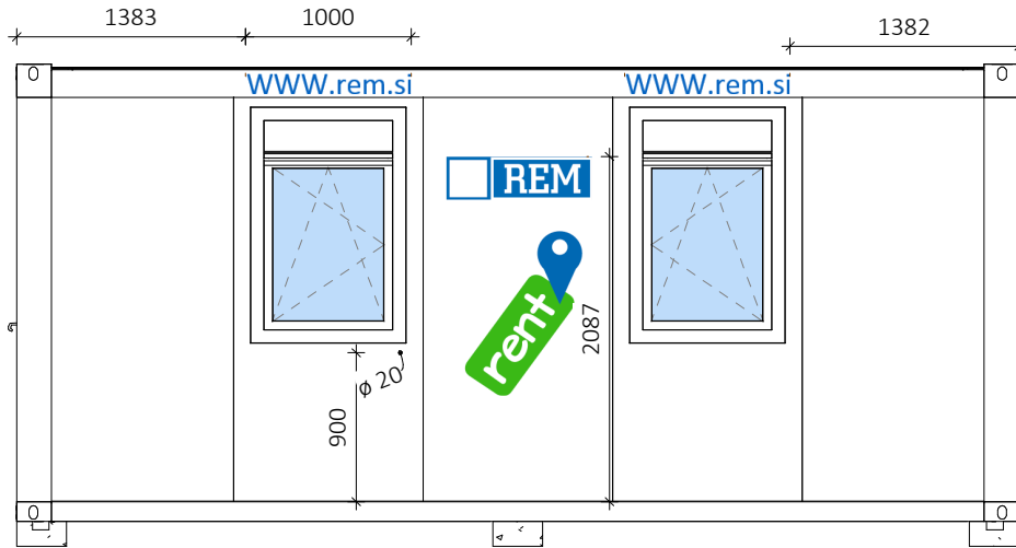
Pogled spredaj 1 : 50
