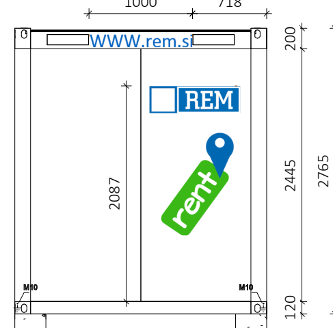
Pogled z desne 1 : 50
