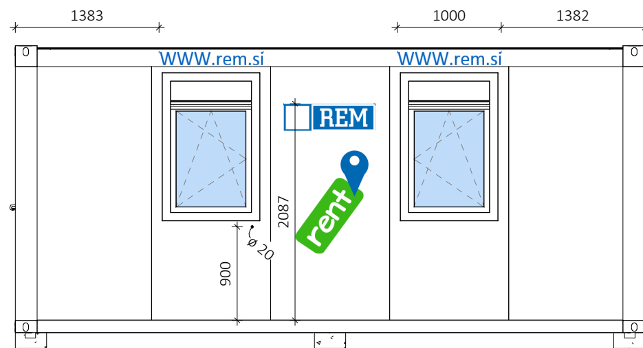
Pogled spredaj 1 : 50
