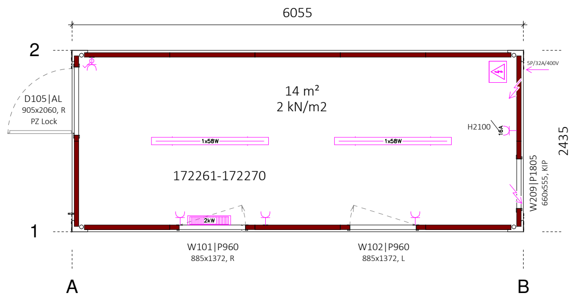
Tloris 1 : 50
