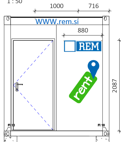
Pogled z leve 1 : 50
