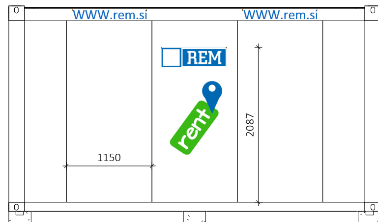
Pogled zadaj 1 : 50
