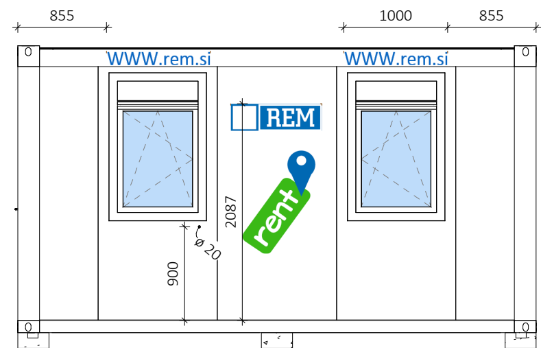
Pogled spredaj 1 : 50
