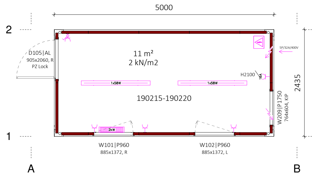
Tloris 1 : 50
