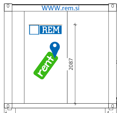
Pogled zadaj 1 : 50
