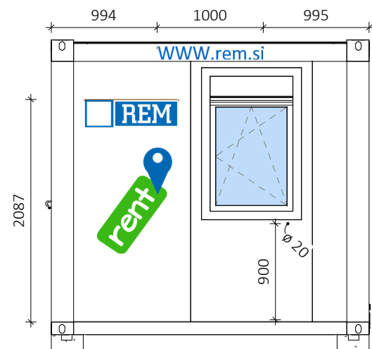
Pogled spredaj 1 : 50
